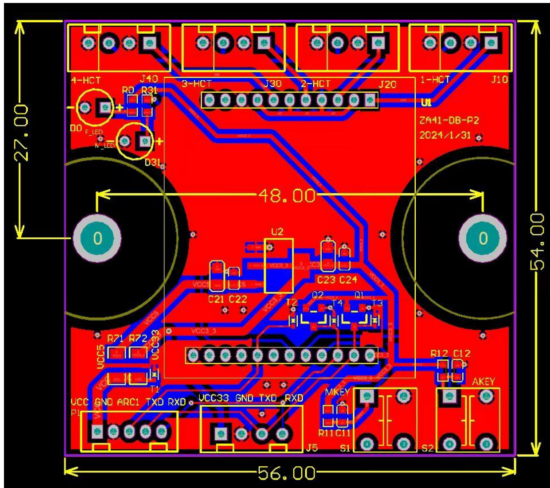
图 1：底板尺寸图(定位孔径为 4.2mm)
