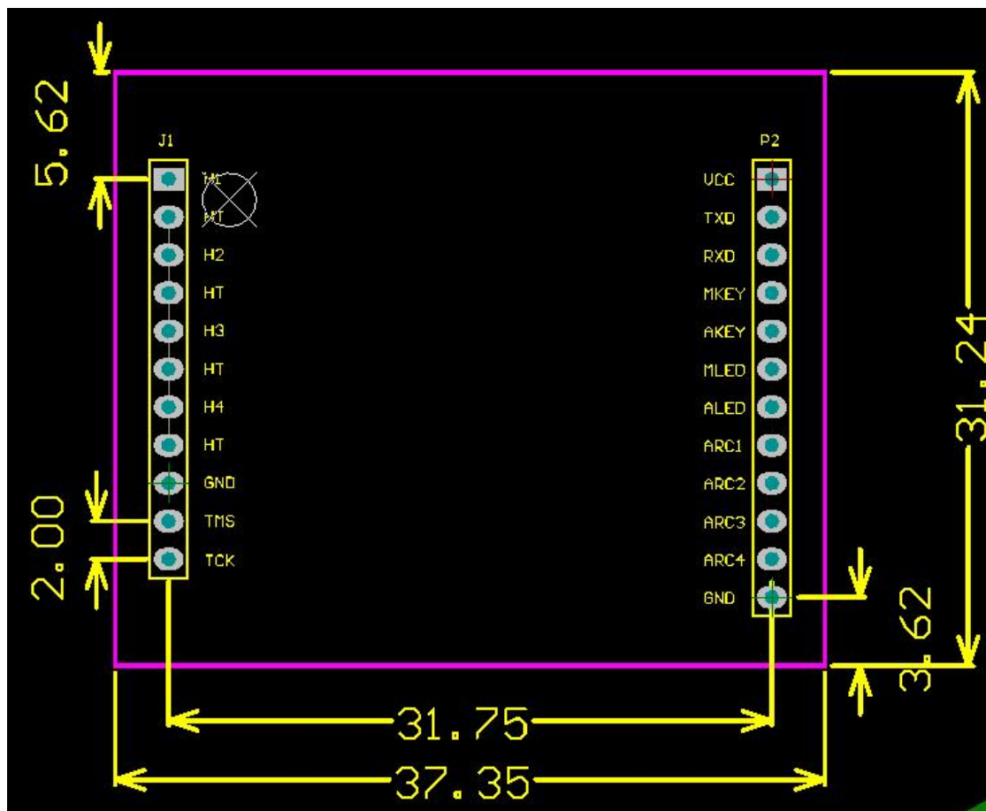
图 2 模组封装尺寸图
